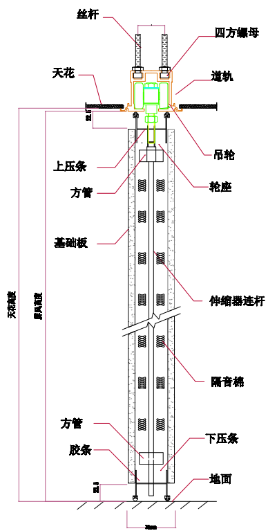
垂直截面
