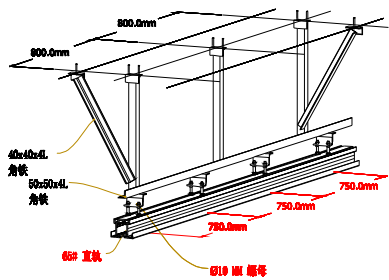
钢结构安装图
