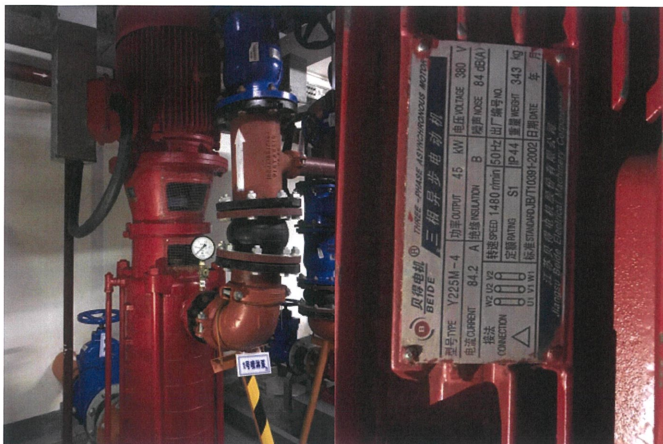
3、稳压泵（三相异步电动机Y112M-2）
