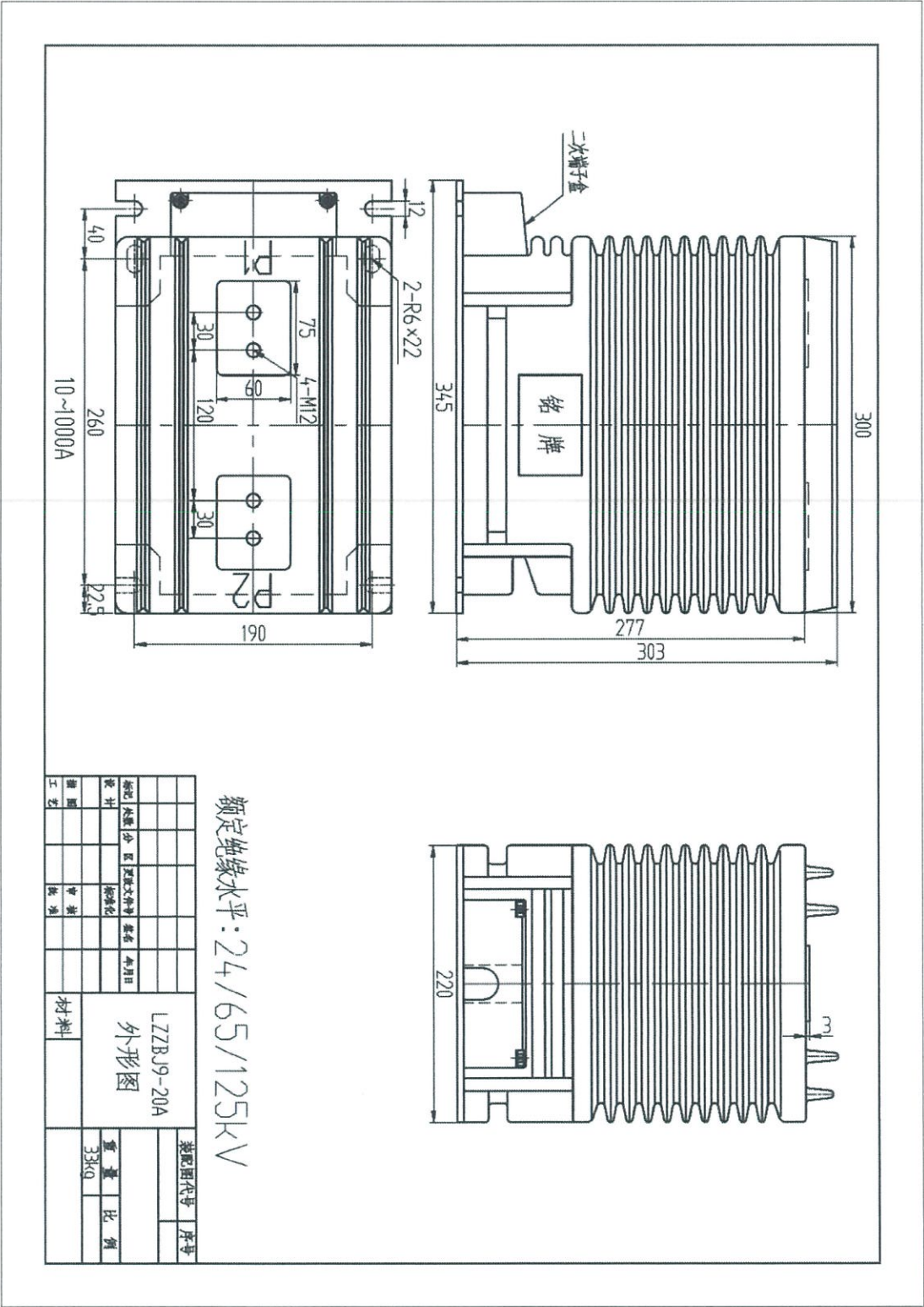
20kV 计量用电流互感器外形图
