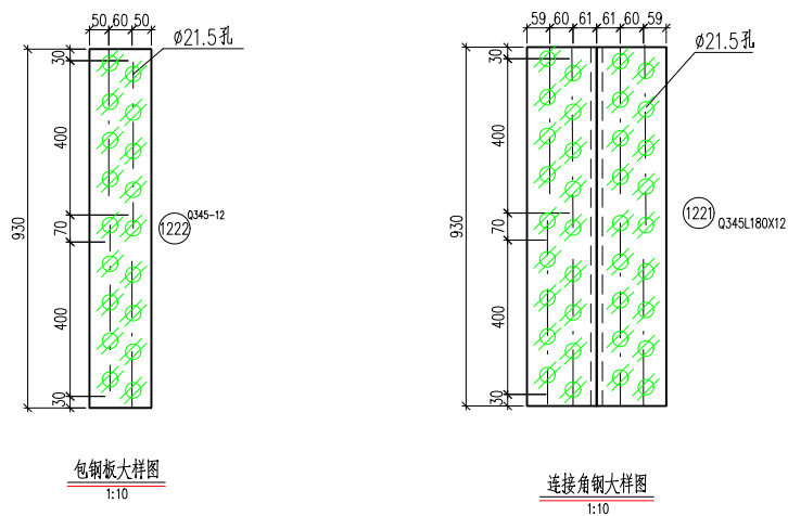
图 4.7 包角钢视图
