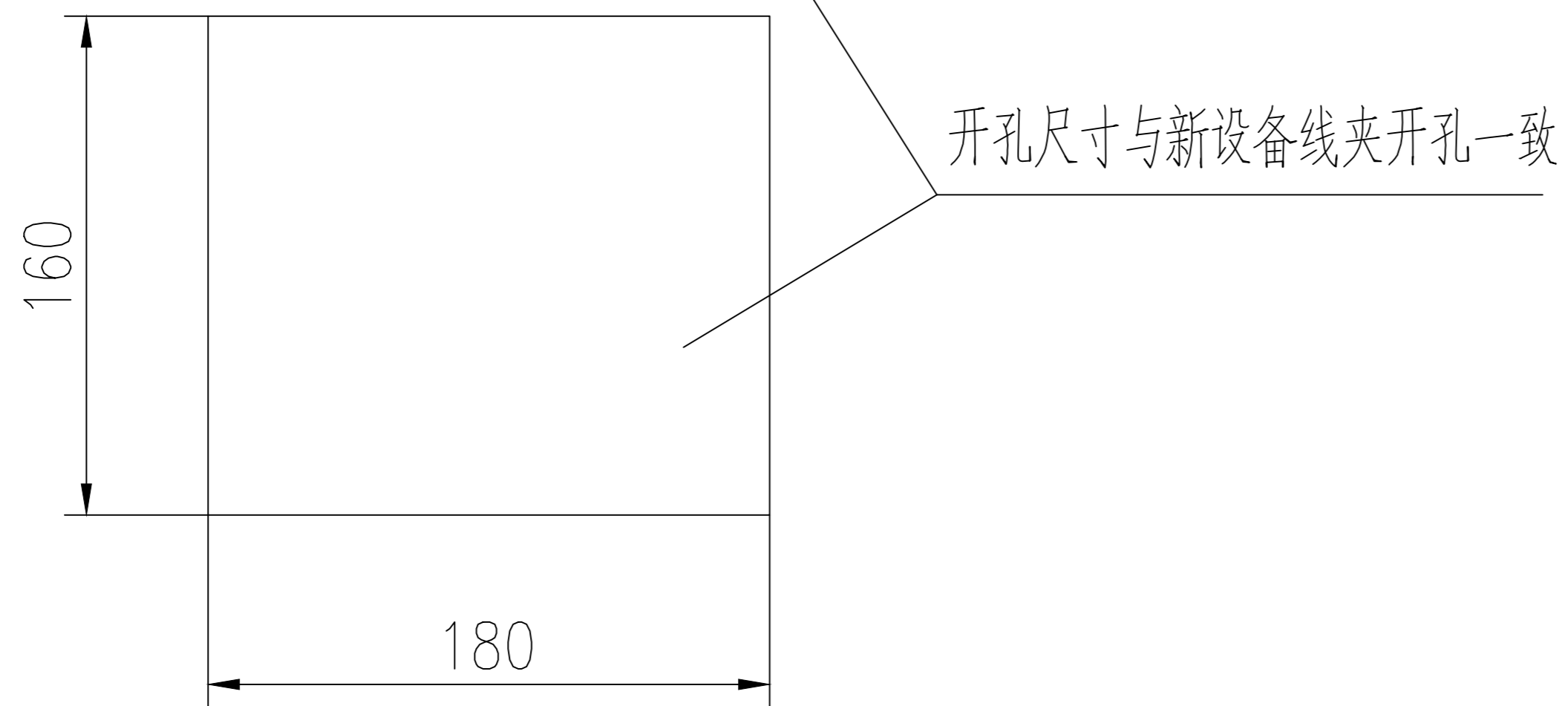
过渡件底板有效接触面积示意图
