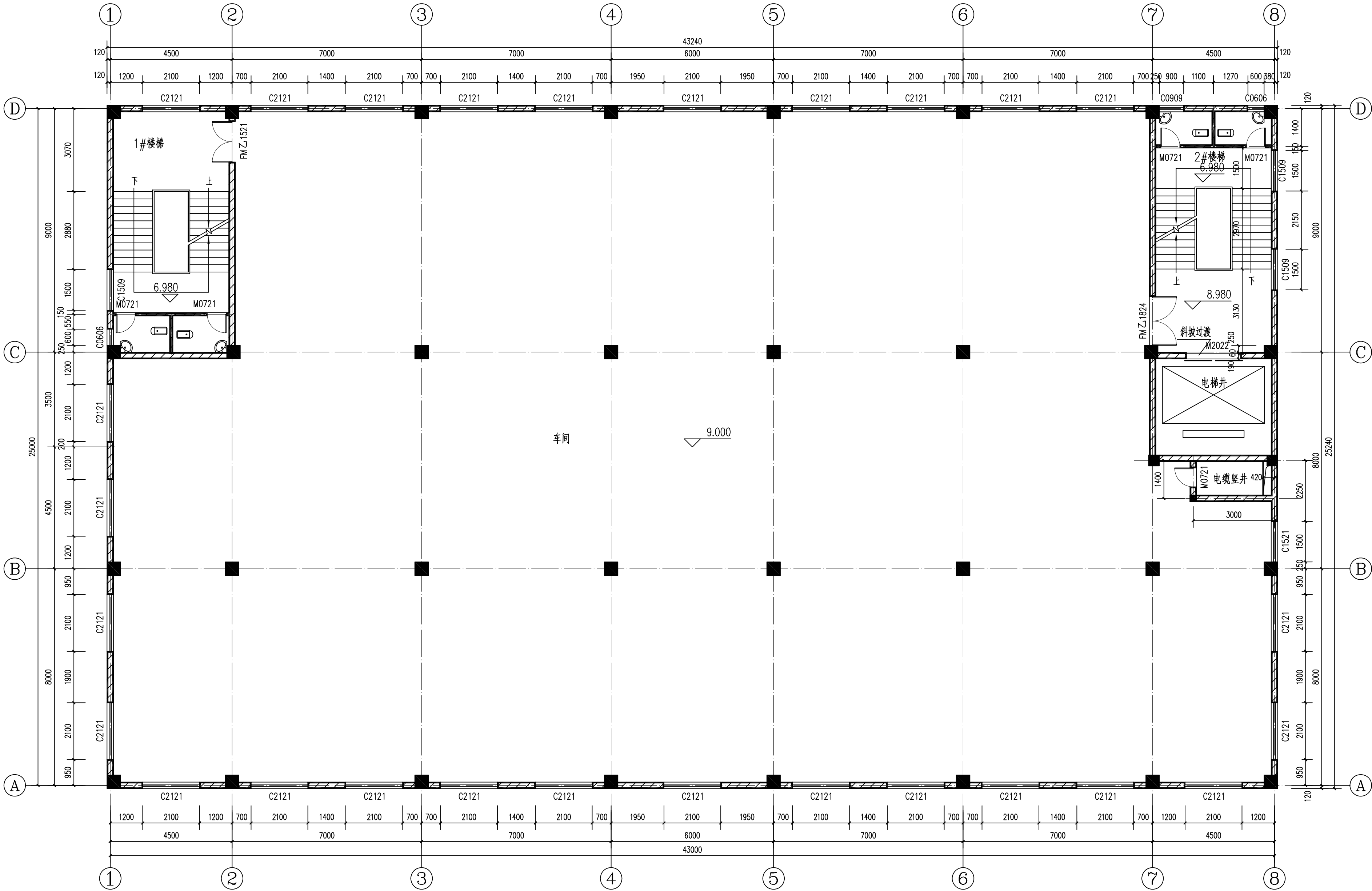
三层平面布置图 1:100
