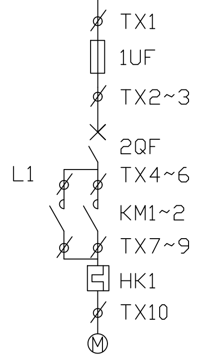
一次方案图
