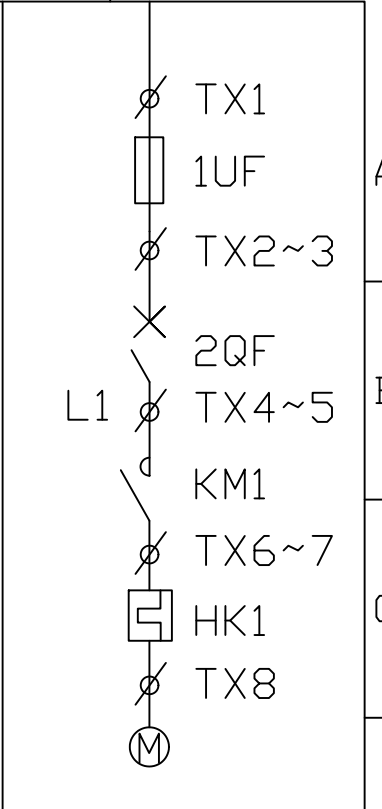
一次方案图
