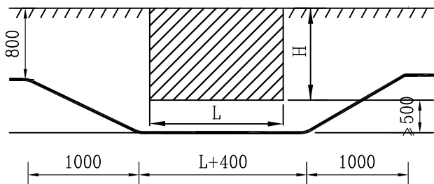
接地线经过道路、建构筑物基础预埋示意
