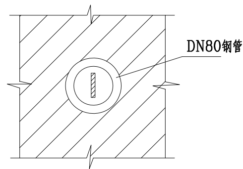
接地线穿墙安装图
