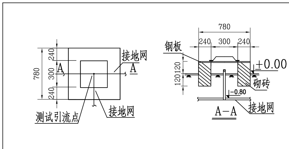
测试引流点制作图
