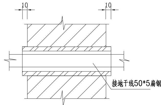
接地线经过电缆沟示意
