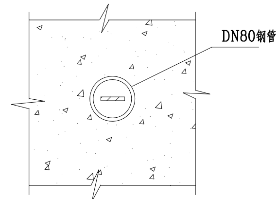
接地线穿楼板安装图
