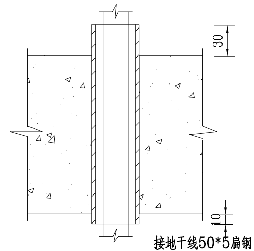
构架引下接地扁钢的连接
