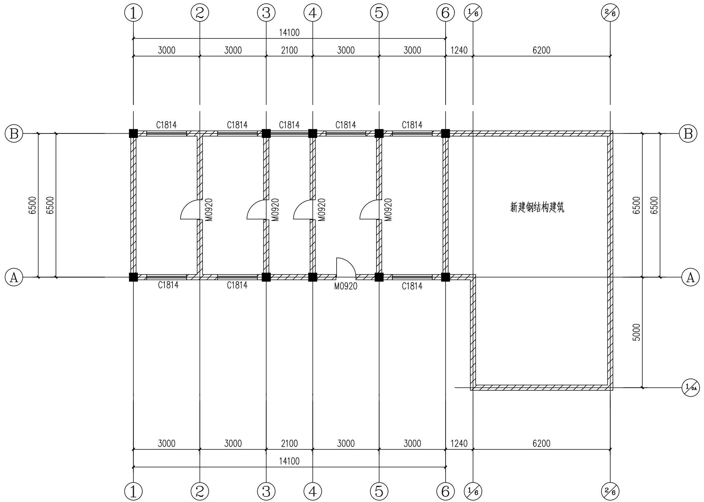
一层平面图 1:100
