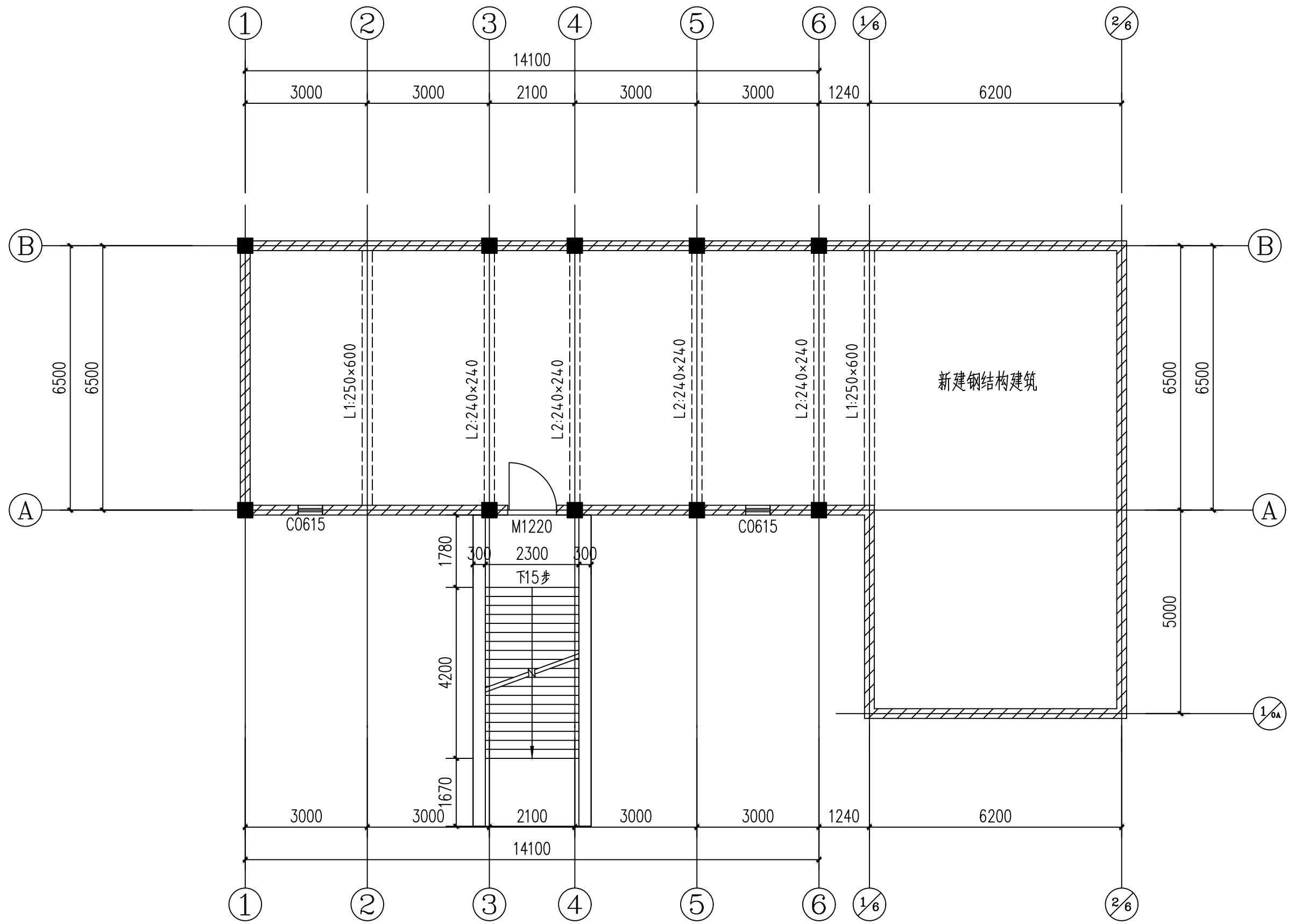
二层平面图 1:100
