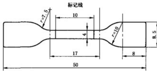
图 13 小哑铃试件
