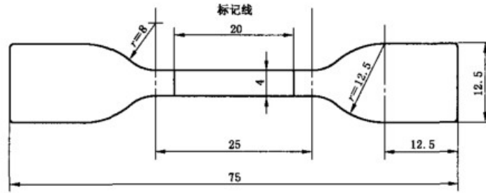
图 12 哑铃试件
