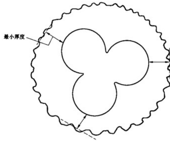
图 9 护套厚度测量(不规整外表面)
