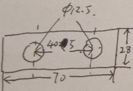
阻尼连接锁片
