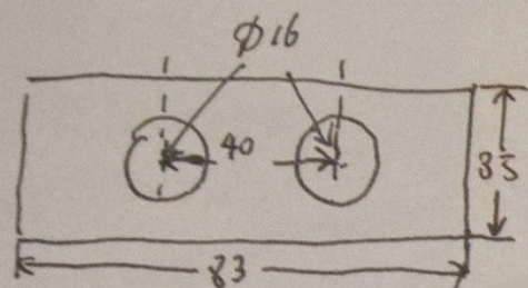
#1. 12 磁极引线锁片
