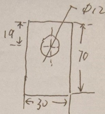
阻尼连接片上下通孔锁片
