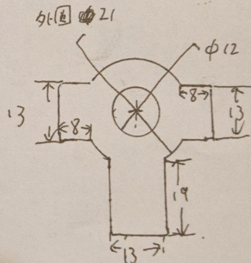
环大牙由铜排 锁片
