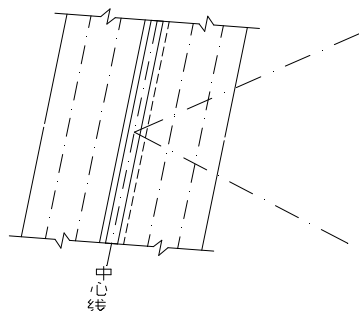
图 4.4 主材为组合角钢构图示意
