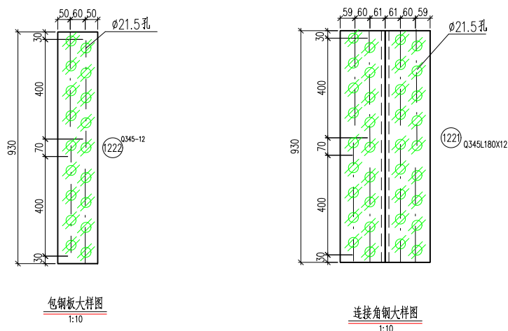
图 4.7 包角钢视图
