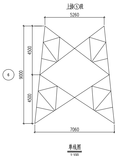
图 3.1 身部单线图
